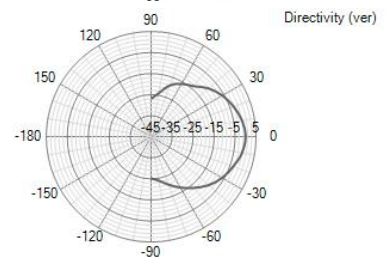
Ver. 8011 Hz, DI=10.5 dB
