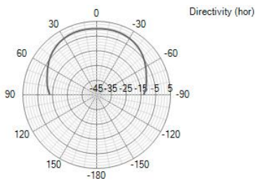
Hor. 2003 Hz, DI=8.8 dB
