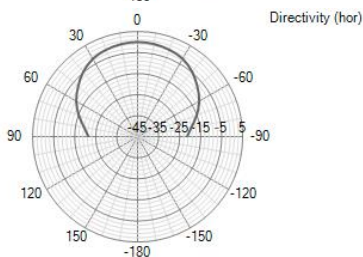
Hor. 8011 Hz, DI=10.5 dB
