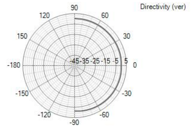
Ver. 125 Hz, DI=3.1 dB
