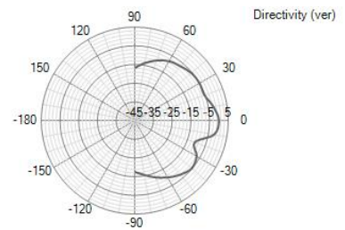
Ver. 2003 Hz, DI=8.8 dB
